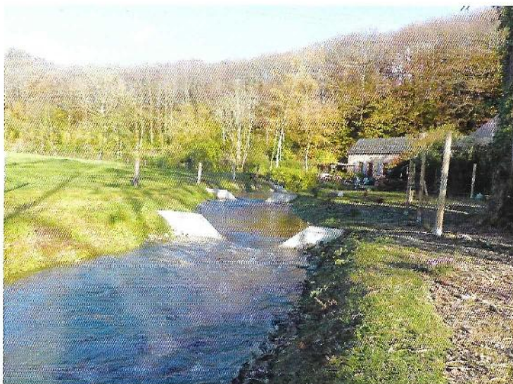
La rivière de contournement du Moulin du David à l'issue des travaux
